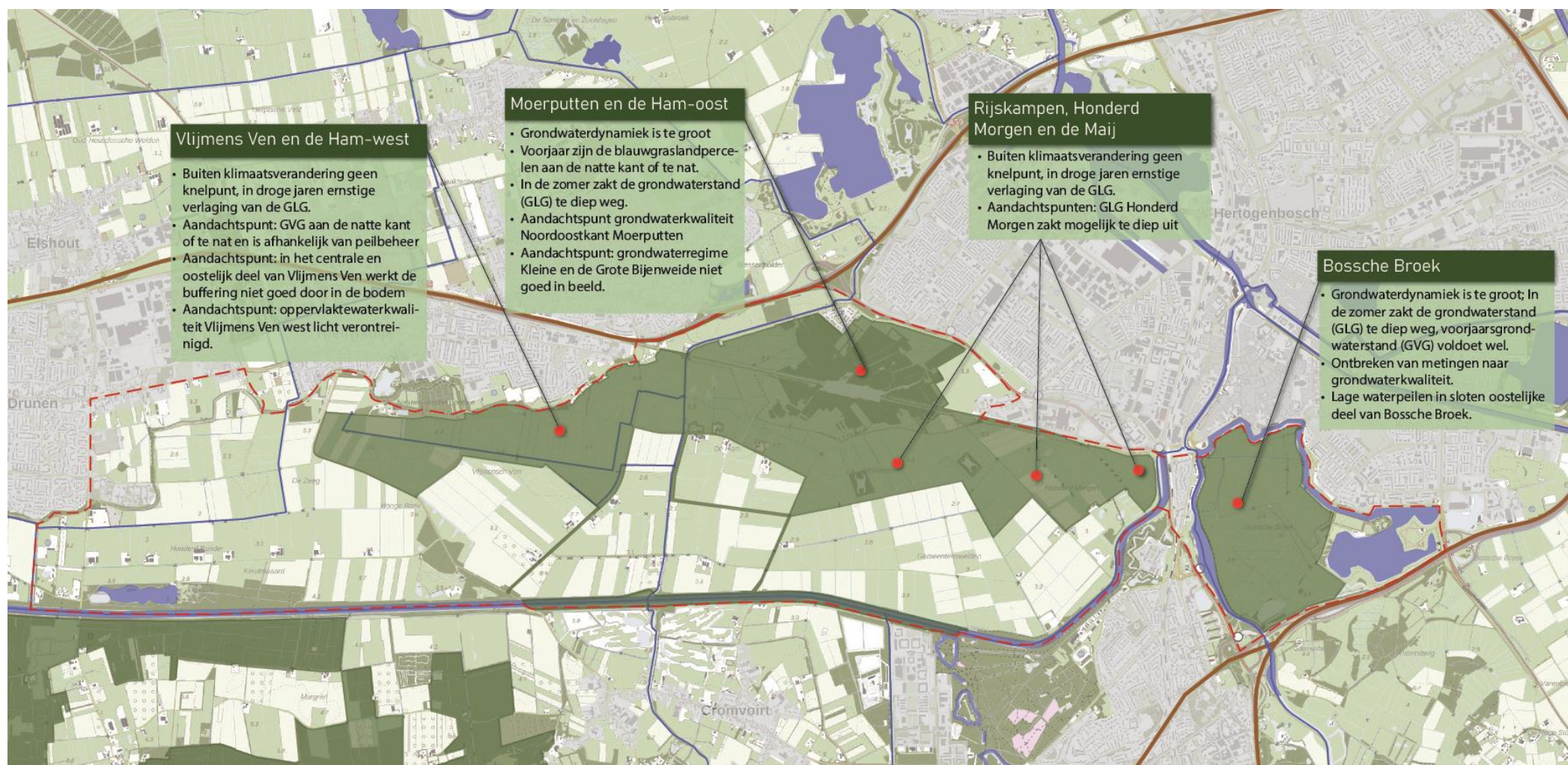
Figuur 204 Conclusies vanuit de EHSA (Ecohydrologische Systeemanalyse). Onder voorbehoud dat effecten van klimaatsverandering niet zijn onderzocht.
