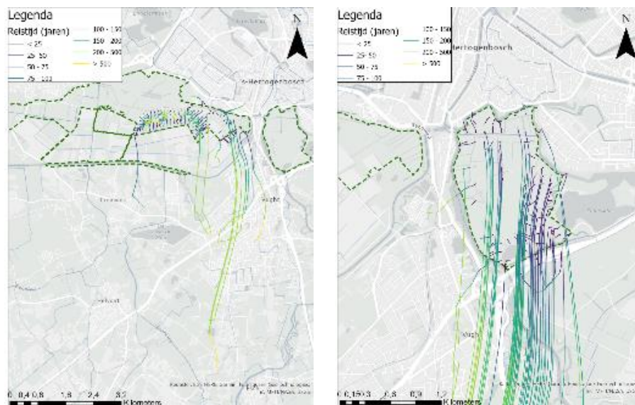
Vervolg Figuur 12 Berekende grondwaterstroombanen vanuit een model (Bron: EHSA 2024 RHDHV)
