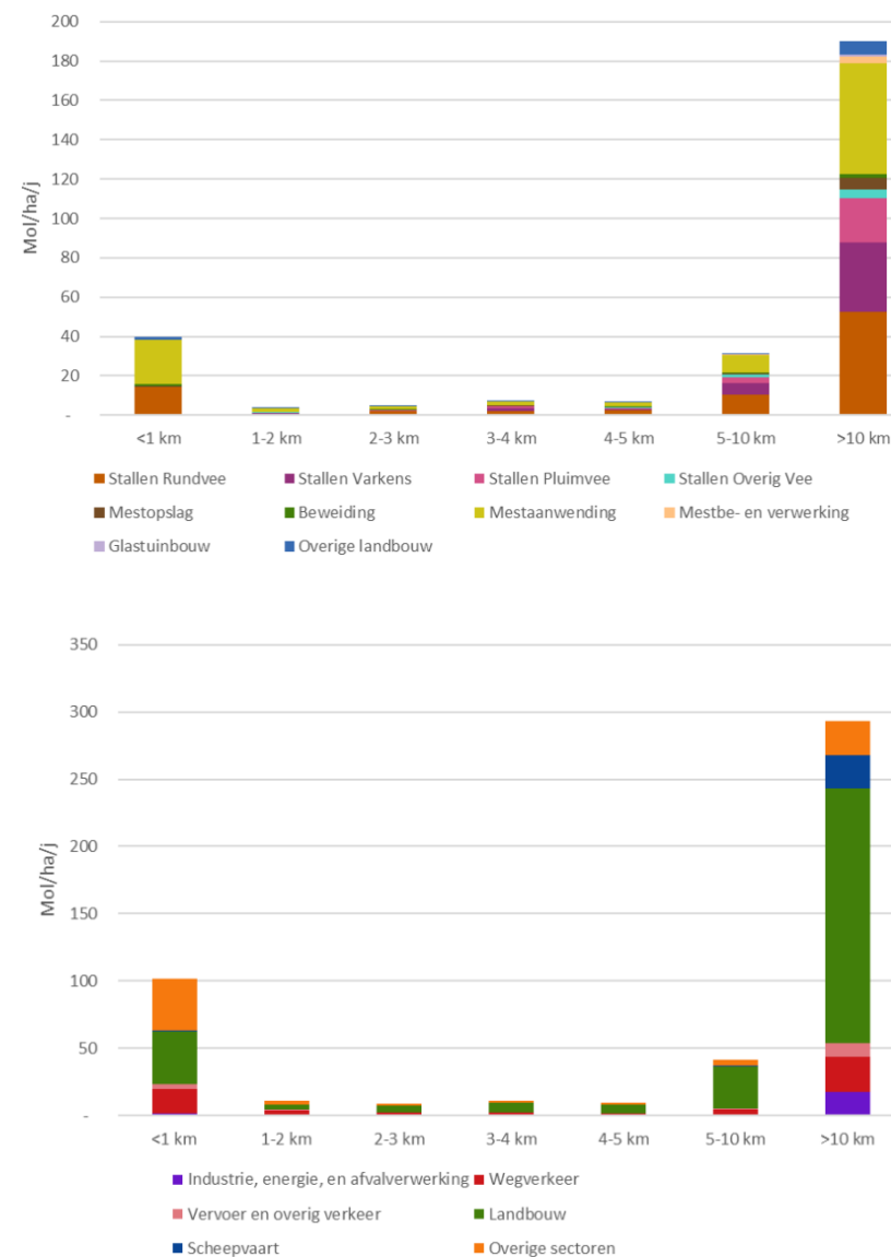
Figuur 24 Nederlandse depositie vanuit bufferzones rondom het N2000-gebied.
