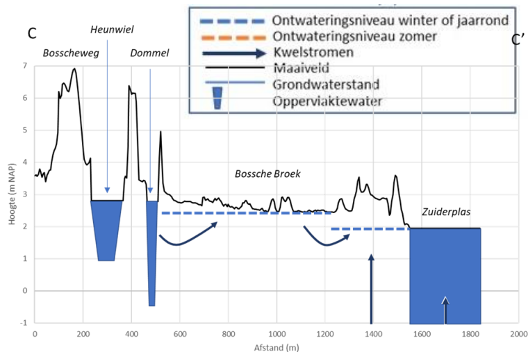
Figuur 11 Grondwaterstroombanen Bossche Broek (Bron: EHSA Vlijmens Ven Moerputten en Bossche Broek 2024 RHDHV)
