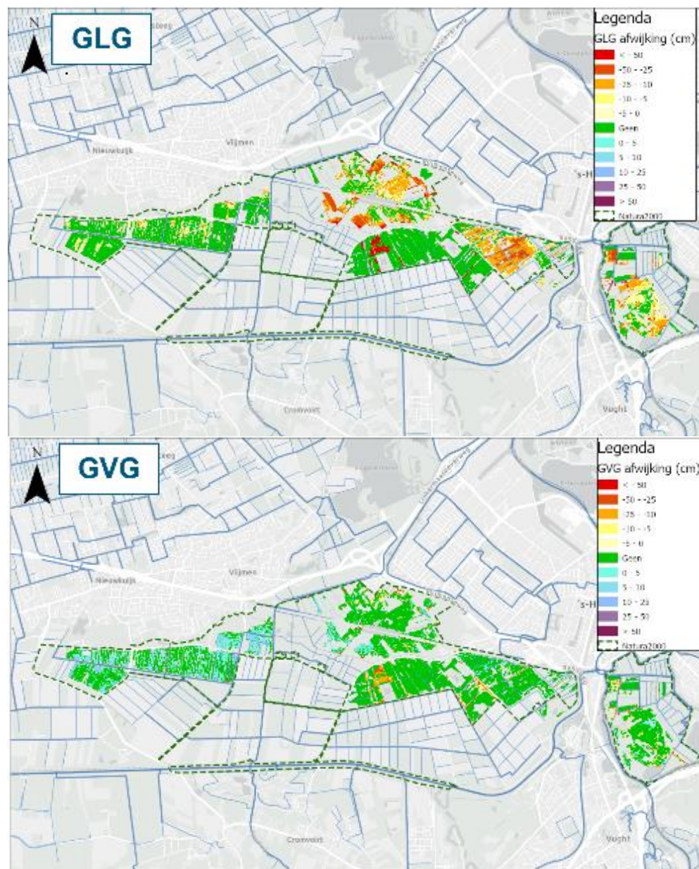
Figuur 21 doelgaten GLG en GVG (EHSA). Een kanttekening bij de kaart over doelgaten GLG is dat model en metingen in Honderd Morgen niet overeenkomen; het oordeel op basis van metingen is dat GLG iets te droog is en dus een minder groot doelgat dan op de kaart. Daarnaast is het effect van droge jaren waarin een extra verlaging van GLG te zien is, hierin niet verbeeld.
