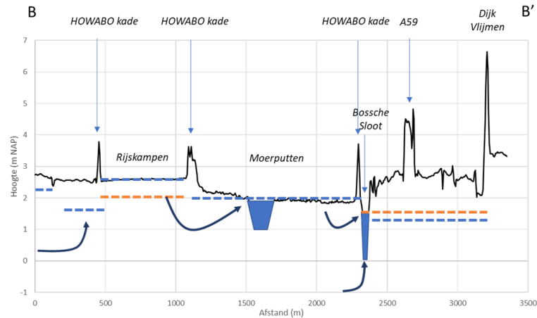
Figuur 10 Grondwaterstroombanen Moerputten, Rijskampen (Bron: EHSA Vlijmens Ven Moerputten en Bossche Broek 2024 RHDHV)
