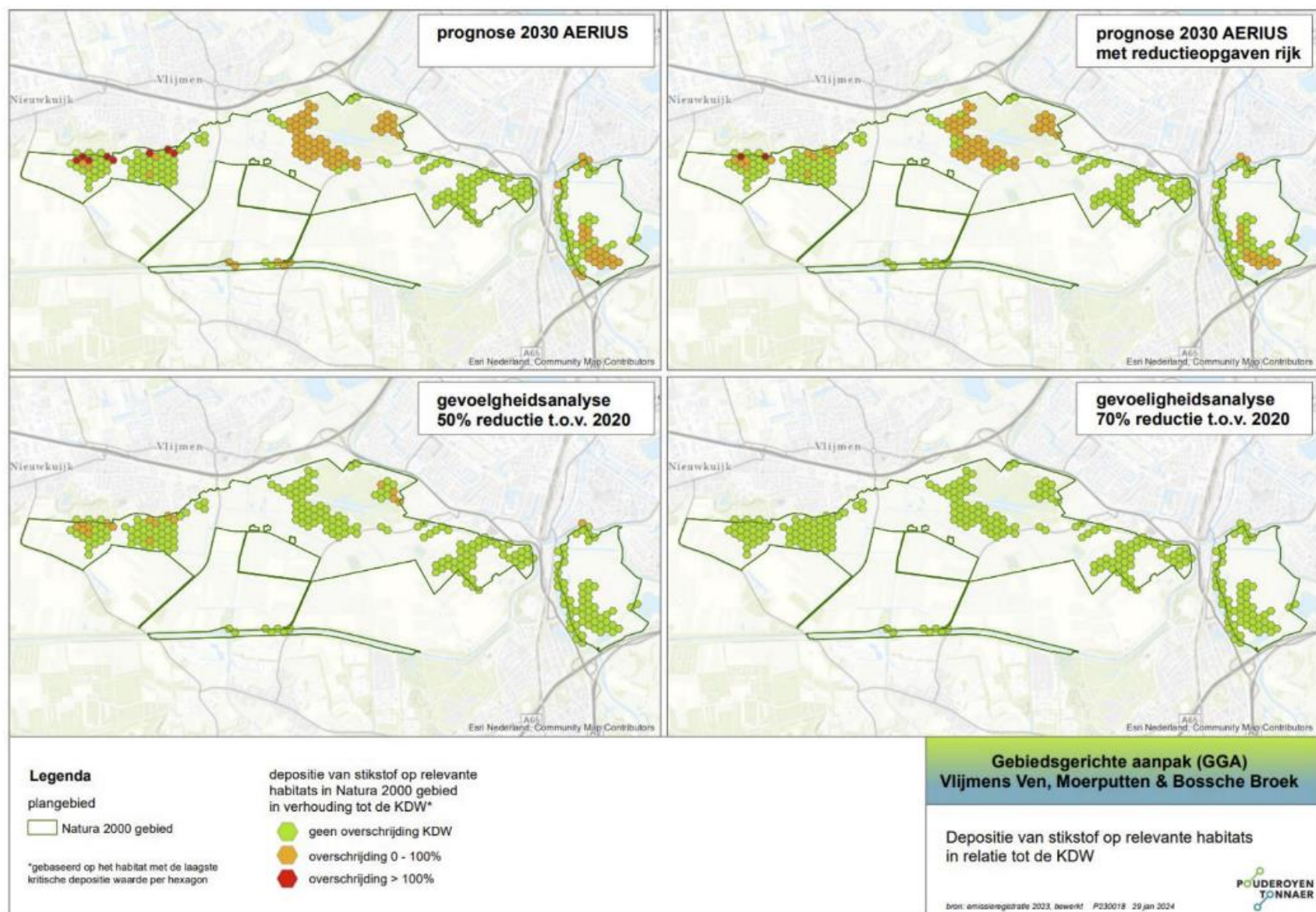
Figuur 25 Depositie van stikstof op relevante habitats in relatie tot de KDW.
