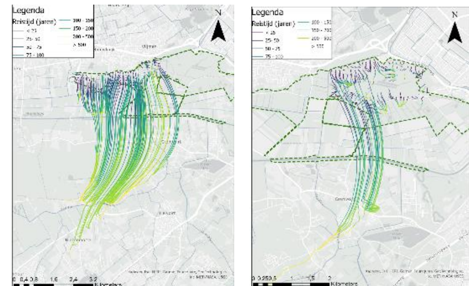
Figuur 12 Berekende grondwaterstroombanen vanuit een model (Bron: EHSA Vlijmens Ven Moerputten en Bossche Broek 2024 RHDHV)
