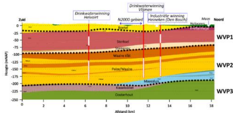
Figuur 5 Doorsnede: geohydrologische opbouw met watervoerende pakketten en waterwinningen (Bron: EHSA 2024 RHDHV)
