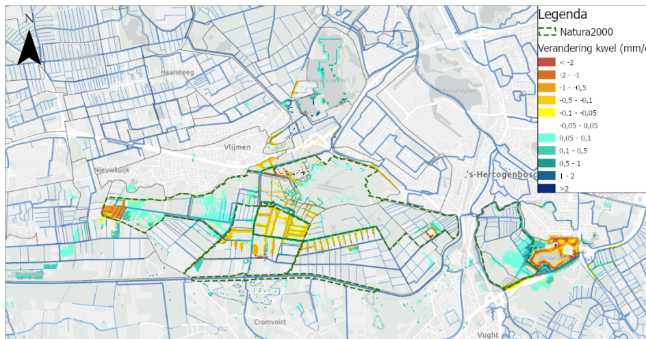
Verandering kwelflux winter maatregelpakket 1 (links) en maatregelpakket 2 (rechts)
