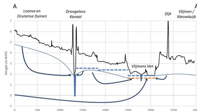
Figuur 9 Grondwaterstroombanen Vlijmens Ven en De Ham (Bron: EHSA Vlijmens Ven Moerputten en Bossche Broek 2024 RHDHV)
