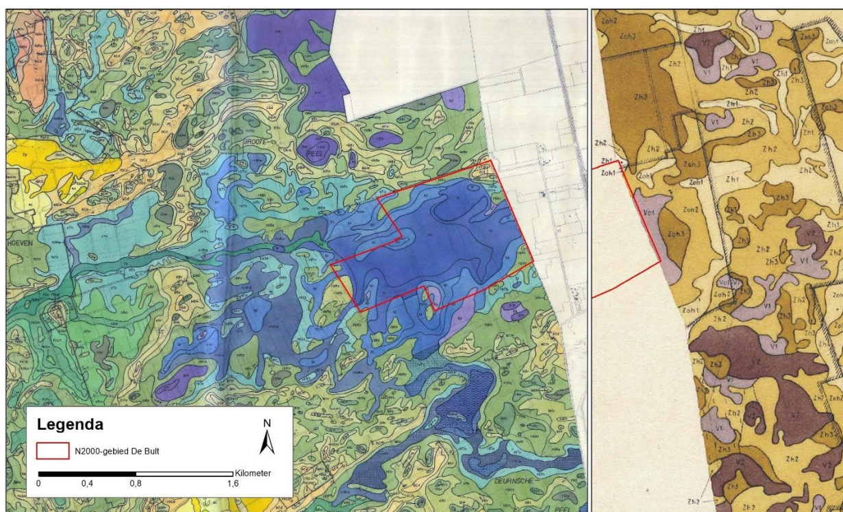
Figuur 3-5: Uitsnede voor De Bult en omgeving uit de gedetailleerde bodemkaarten Brabantse Peel (links) en Venray (rechts) uit 1955 (Ceelen & Kanter 1955; van Nispen tot Pannerden 1955).
