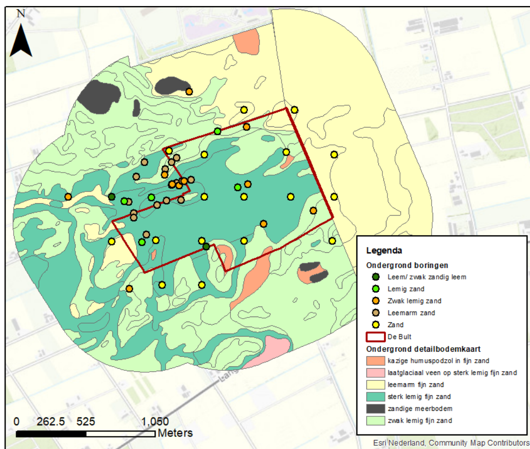
Figuur 3-8: Ondergrond uit de detailbodemaart en uit de beschikbare boringen (boorbeschrijvingen beschikbaar gesteld door Waterschap Aa en Maas (Kiestra 2017), en uit (Dinoloket 2022).
