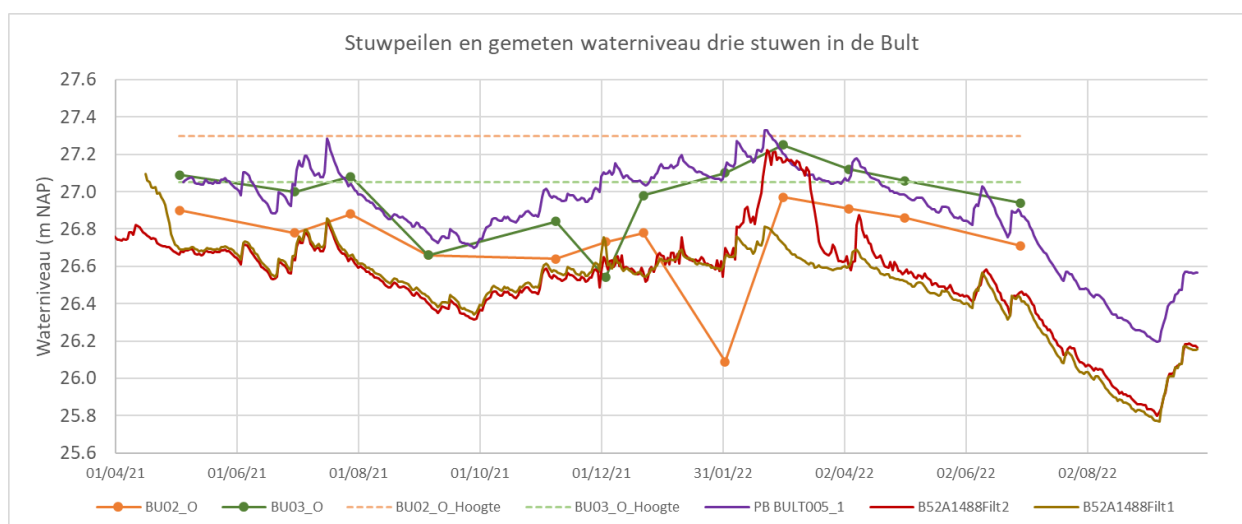
Figuur 3-22: Tijdreeksen van de gemeten waterstanden bij de stuwen, de ingestelde stuwstanden en de gemeten stijghoogte in B52A1488 en BULT005. *Meting in BU02_O van januari 2022 lijkt een meetfout.
