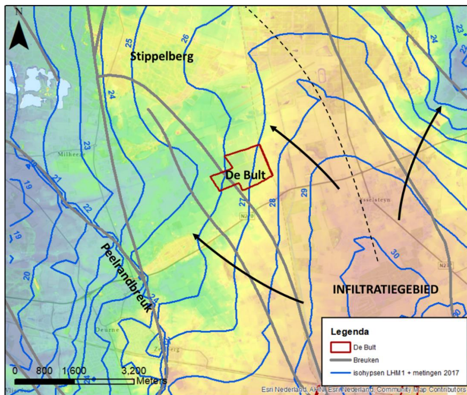
Figuur 3-12: Isohypsen LHM1 (+metingen uit 2017) (Bron: (Grondwatertools 2022)). De zwarte onderbroken lijn geeft globaal de ligging van de waterscheiding aan.
