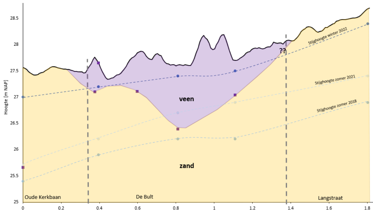
Figuur 3-35 Noord-Zuid dwarsdoorsnede oostelijk deel door de Bult (zoals weergegeven in Figuur 3-34) met daarin weergegeven het maaiveld, indicatie veenlaag (paarse vlak, vierkantjes geven onderkant veen in boring weer) en gemeten stijghoogte.
