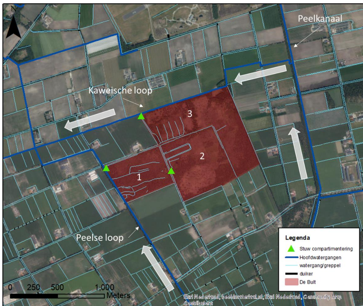
Figuur 3-26: Oppervlaktewatersysteem in de omgeving van De Bult.
