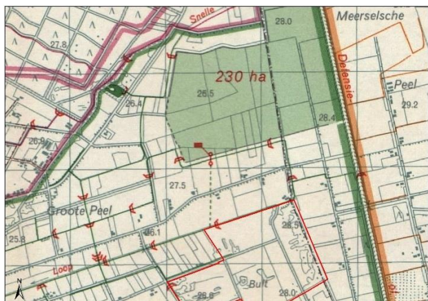
Figuur 3-14: Bemalingsgebied Vliegbasis De Peel (linker afbeelding) volgens Waterstaatskaart 5 e editie 52 Venlo West 1 uit 1986 (Rijkswaterstaat 2022). In rood de begrenzing van De Bult. De foto (11 oktober 2022) rechts laat het verval zien over een stuw 261JB aan de Koperenpeel stroomafwaarts van dit bemalingsgebied.
