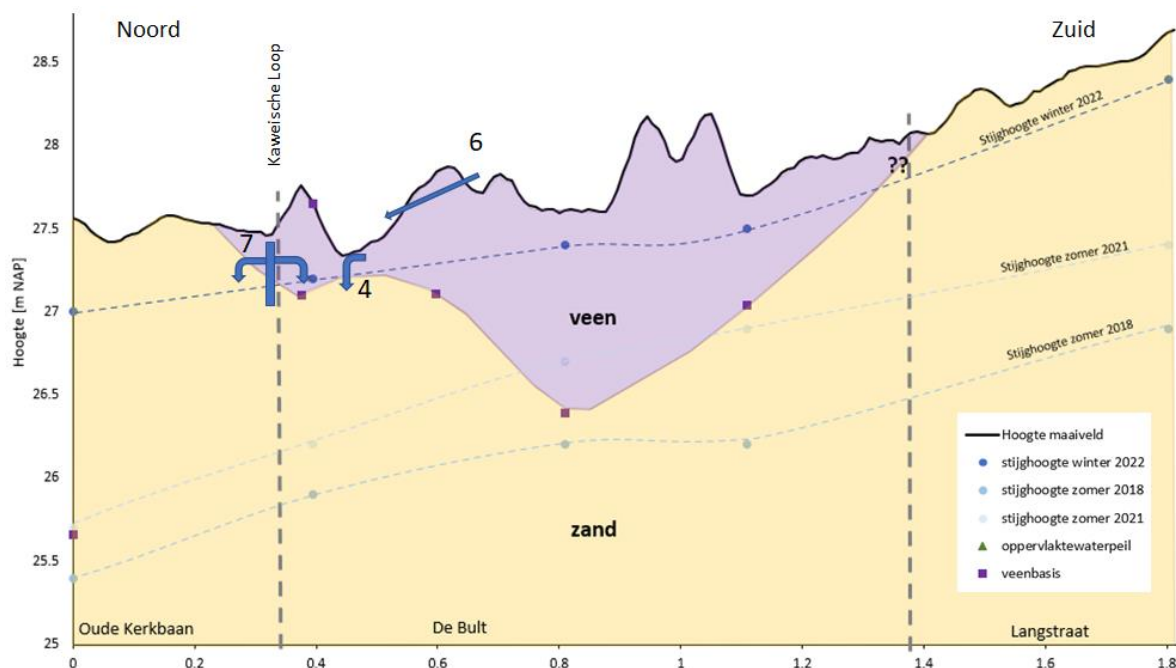
Figuur 4-22 Schematische bodemopbouw op noord-zuid doorsnede door De Bult (oostelijke deel). Maaiveld o.b.v. AHN4 en veendikte op basis van boringen en detail bodemkaart. Op de doorsnede zijn de verschillende manieren weergegeven waarop (grond)water het gebied kan verlaten (pijlen met nummering).
